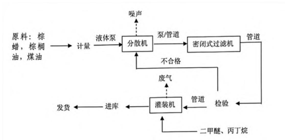
图 4.1-1 自喷蜡分装生产工艺流程图
