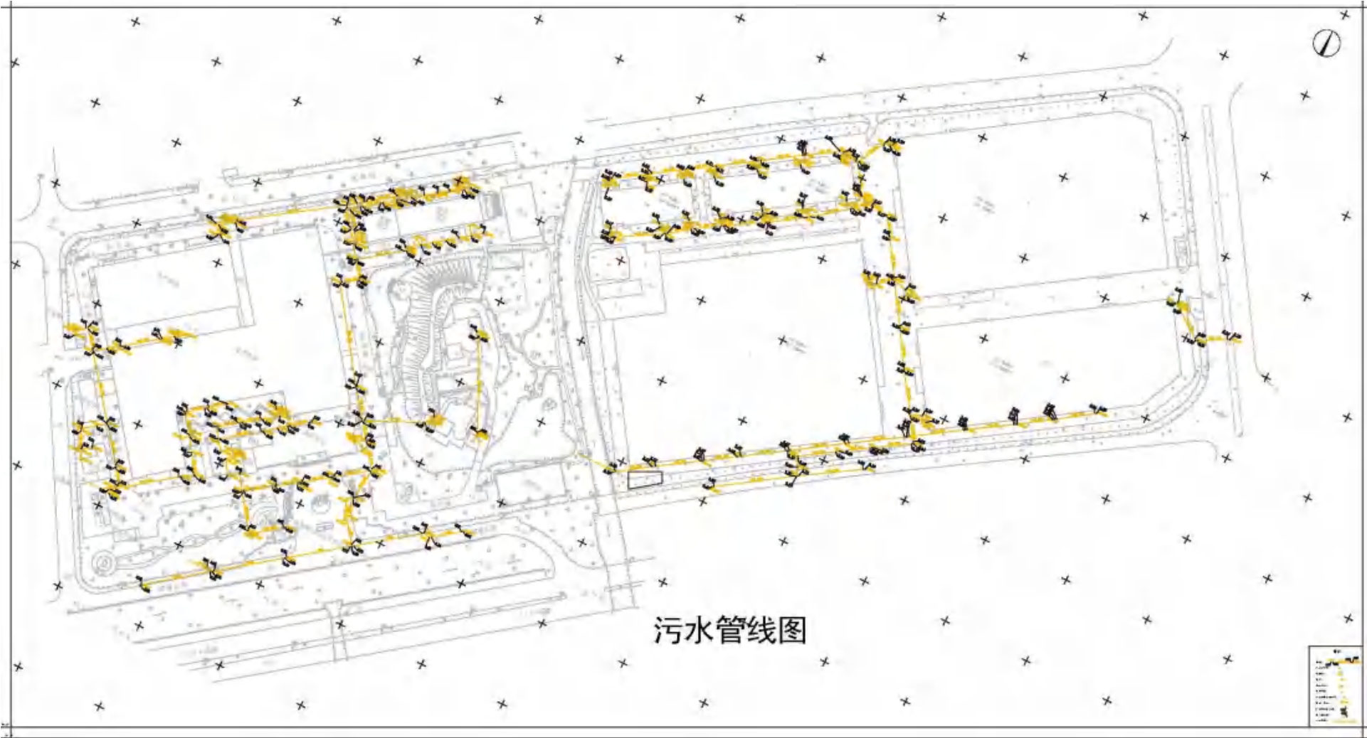
图 4.2-2 厂区污水管网分布图
