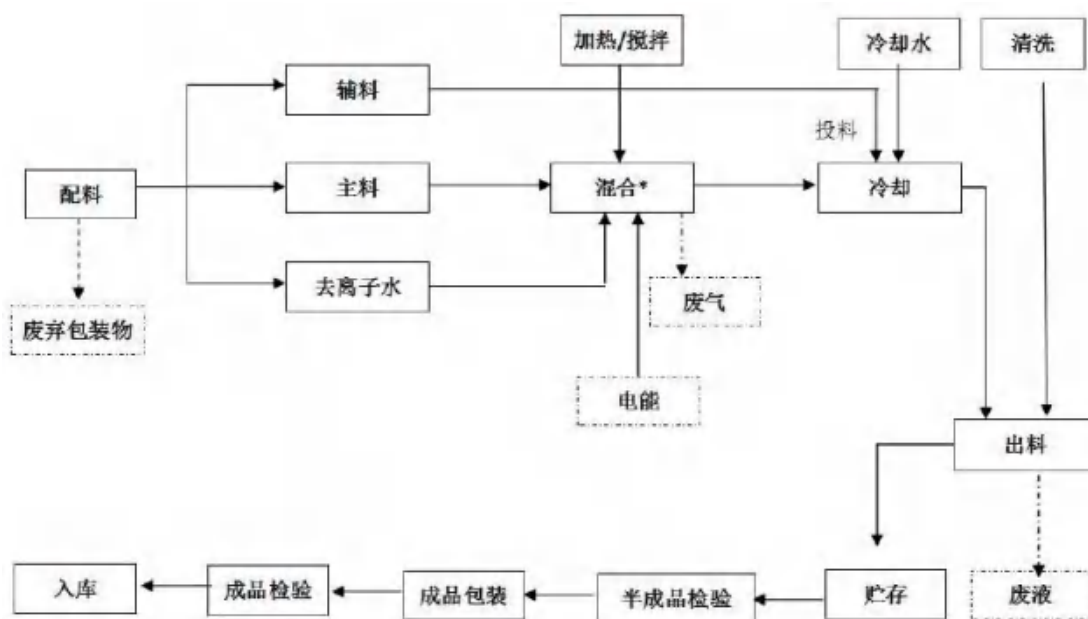
4.1-12 一般液态单元生产工艺流程图
