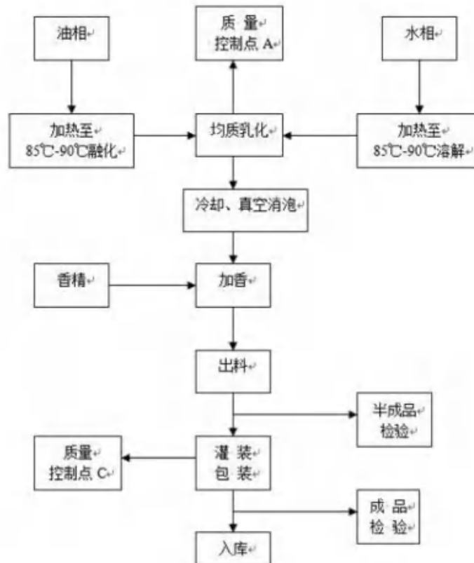
图 4.1-3 护肤（乳液）生产工艺流程图
