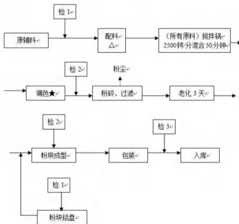
图 4.1-1 粉类（散粉、块状粉）生产工艺流程图
