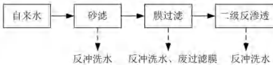
图 4.1-7 纯水工艺流程图
