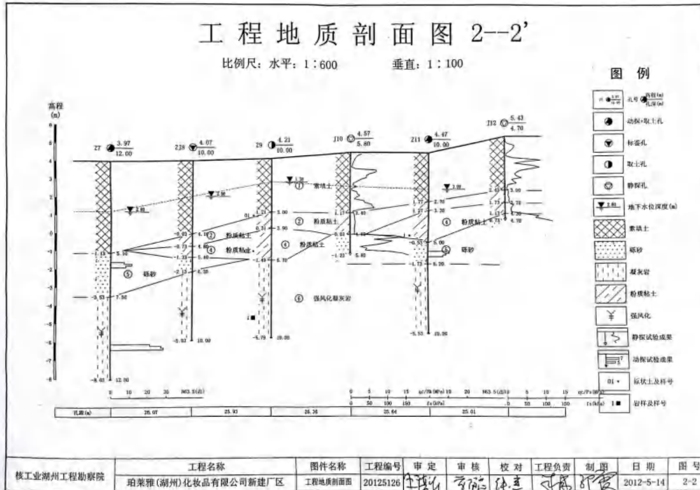
图 3.1-6 三期工程地质剖面图
