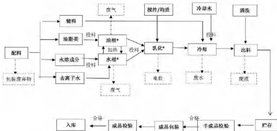
4.1-11 膏霜乳液单元生产工艺流程图
